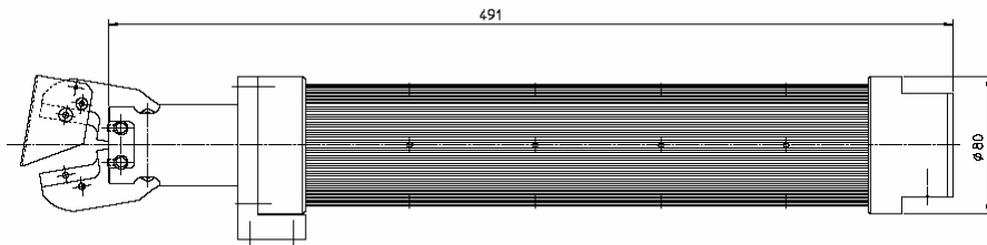
Zangenkörper: Länge 491 mm Durchmesser \varnothing 80 mm
