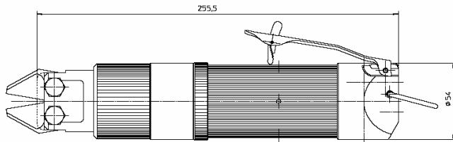
Zangenkörper: Länge 255,5 mm Durchmesser Ø54 mm
