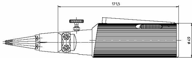
Zangenkörper: Länge 1715 mm Durchmesser ø49 mm
