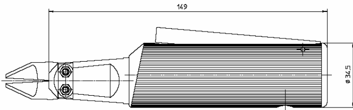
Zangenkörper: Länge 149 mm Durchmesser 34,5 mm
