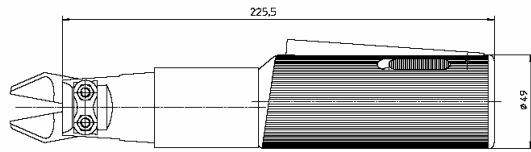
Zangenkörper: Länge 225,5 mm Durchmesser \varnothing 49 mm
