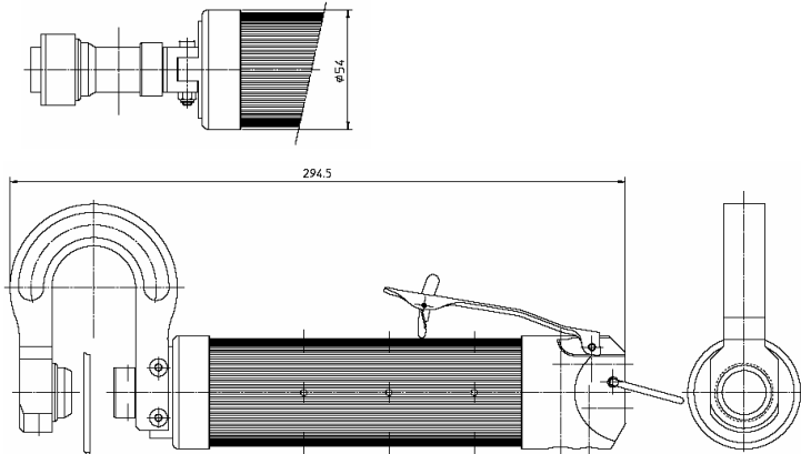
Zangenkörper (incl. Kopf): Länge 294,5 mm Durchmesser \varnothing 54 mm
