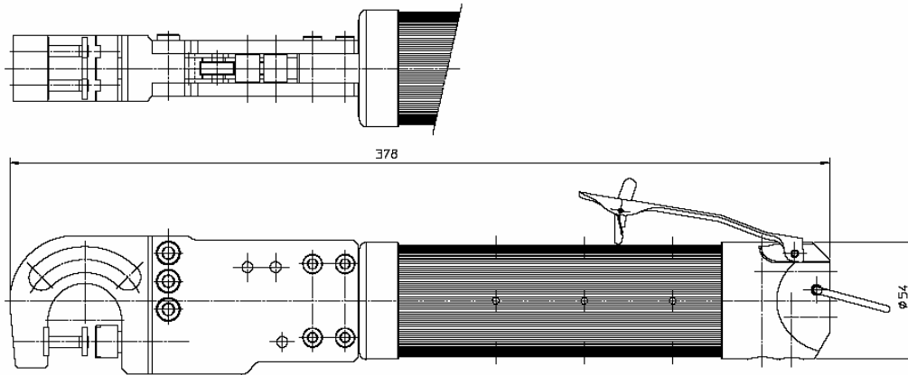
Zangenkörper (incl. Kopf): Länge 378 mm Durchmesser \varnothing 54 mm
