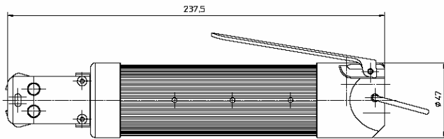
Zangenkörper: Länge 237,5 mm Durchmesser 47 mm
