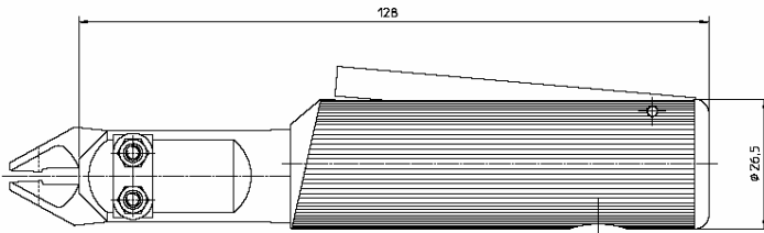
Zangenkörper: Länge 128 mm Durchmesser 26,5 mm
