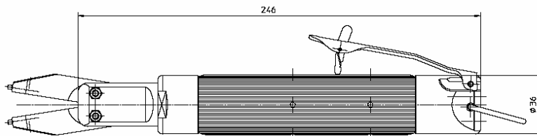
Zangenkörper: Länge 246 mm Durchmesser ø36 mm
