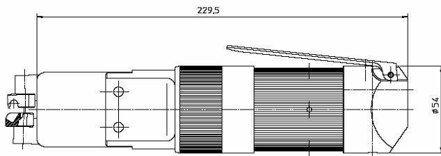
Zangenkörper: Länge 229,5 mm Durchmesser Ø54 mm
