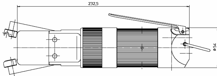
Zangenkörper: Länge 232,5 mm Durchmesser Ø54 mm
