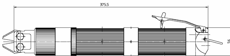
Zangenkörper: Länge 375,5 mm Durchmesser Ø54 mm
