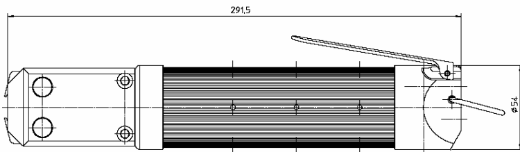
Zangenkörper: Länge 291,5 mm Durchmesser 54 mm
