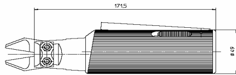
Zangenkörper: Länge 171,5 mm Durchmesser \varnothing 49 mm
