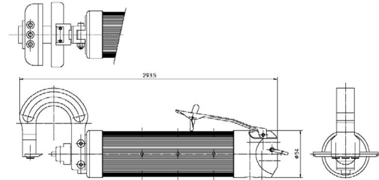
Zangenkörper (incl. Kopf): Länge 293,5 mm Durchmesser \varnothing 54 mm
