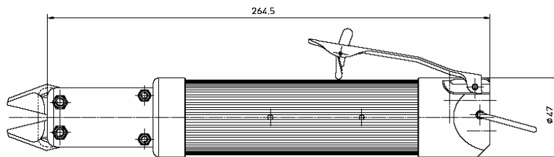
Zangenkörper: Länge 264.5 mm Durchmesser \varnothing 47 mm
