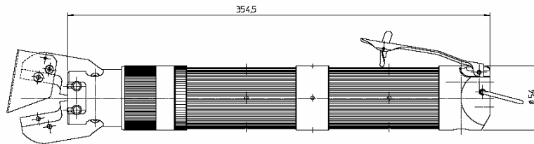
Zangenkörper: Länge 354,5 mm Durchmesser \varnothing 54 mm
