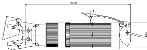
Zangenkörper: Länge 234,5 mm Durchmesser \varnothing 54 mm
