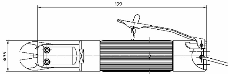
Zangenkörper: Länge 199 mm Durchmesser \varnothing 36 mm
